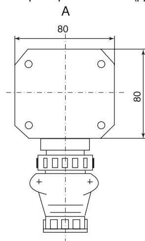
Первичный преобразователь (датчик)
