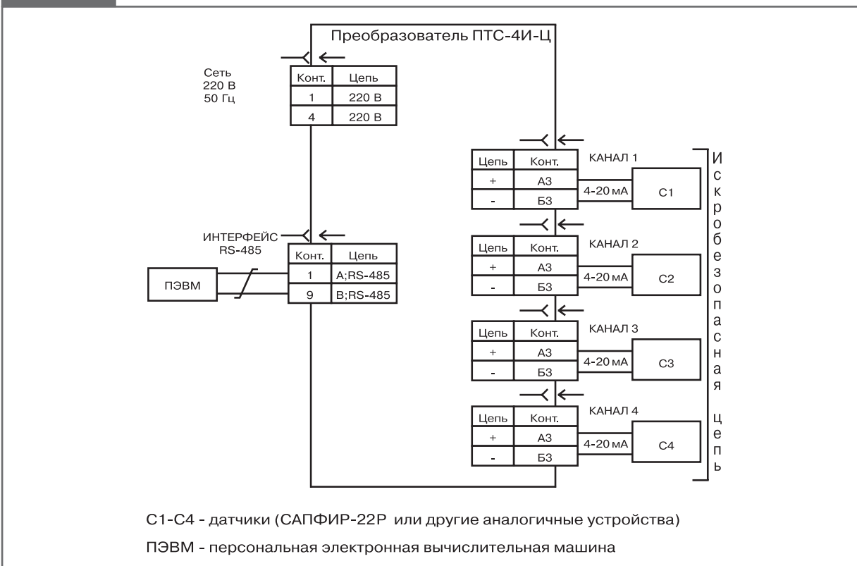
Схема подключения преобразователя ПТС-4И-Ц.
