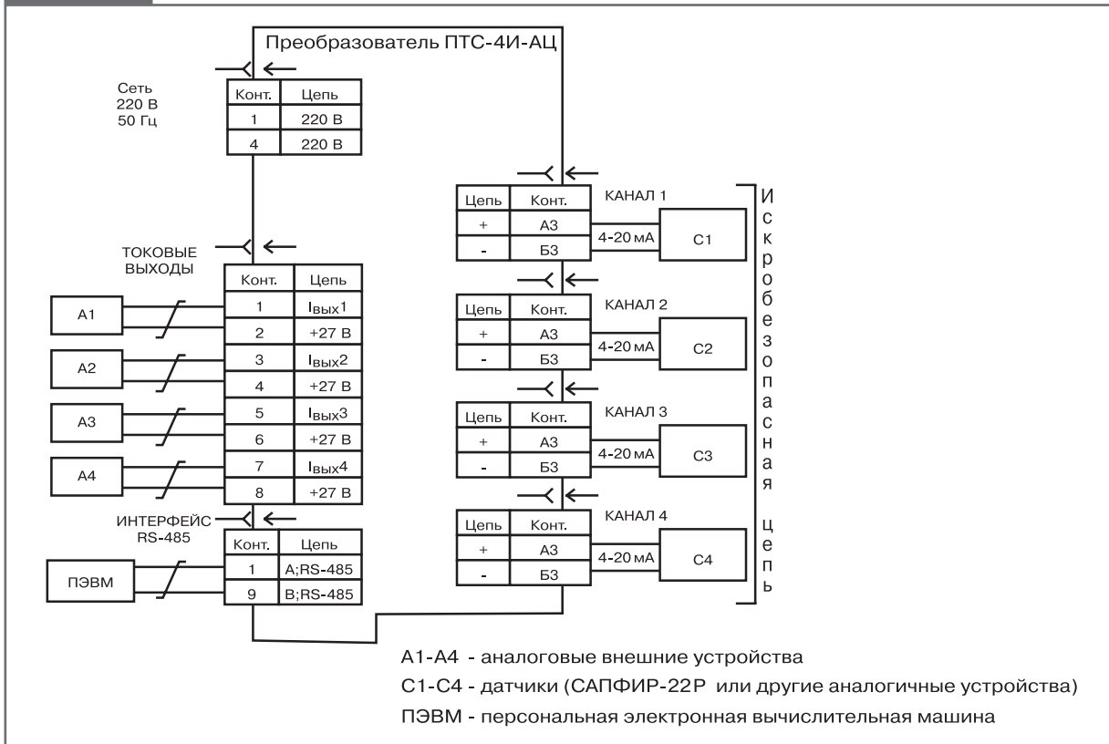
Схема подключения преобразователя ПТС-4И-АЦ.
